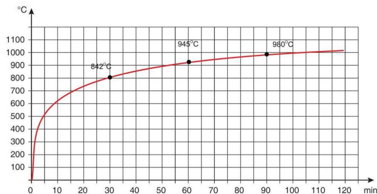
Rys. 4 Krzywa narastania temperatury obrazująca pożary celulozowe[10]
