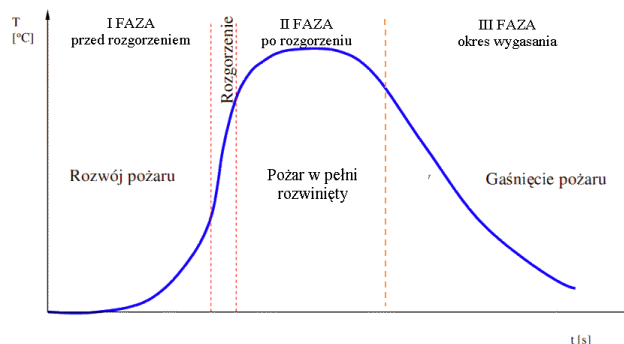
Rys. 2 Krzywa rozwoju pożaru w pomieszczeniu – średnia temperatura pożaru w funkcji czasu.
