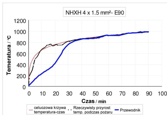
Rys. 7 Przebieg czasowy nagrzewania się izolacji oraz żyły miedzianej przewodu czterożyłowego [18]
