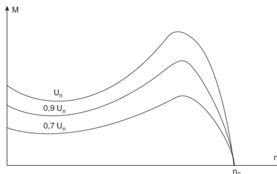
Rys. 9.: Charakterystyki momentu obrotowego silnika indukcyjnego klatkowego dla różnych wartości napięcia zasilającego [19]
