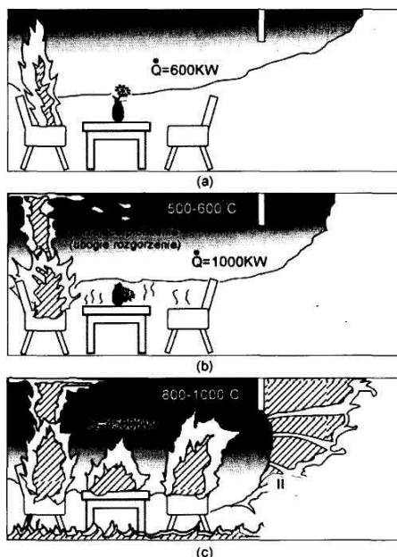
Rys.3 Ogólny obraz I i II fazy pożaru w pomieszczeniu [13; 12]
