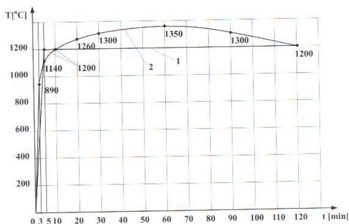
Rys. 5 Krzywe tunelowe „temperatura – czas” [17]
