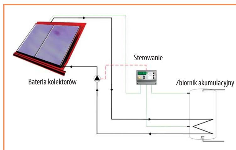
Rys. 11. Sterowanie systemem z obiegiem wymuszonym
