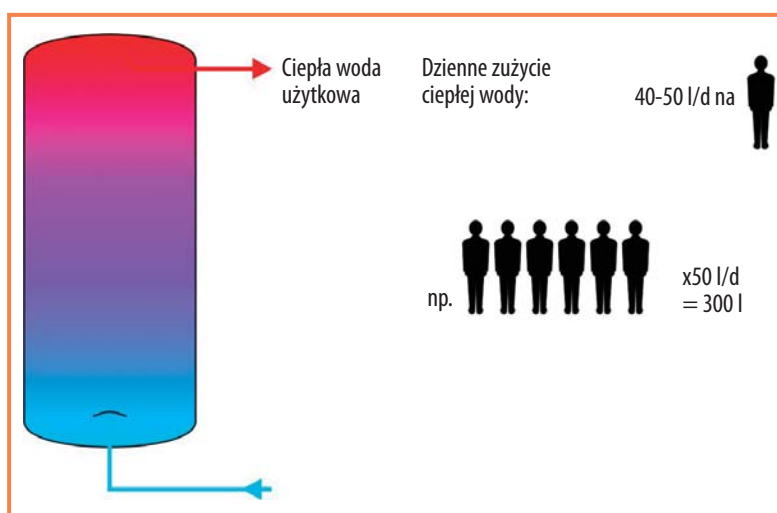
Rys. 18. Wymiarowanie zbiornika akumulacyjnego
