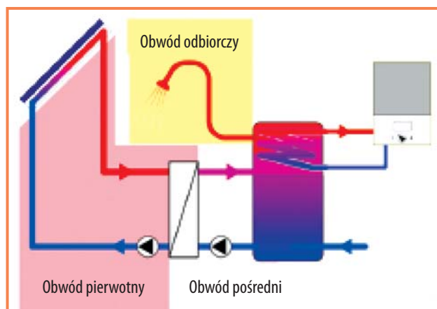
Rys. 10. Obwód pierwotny z zewnętrznym wymiennikiem ciepła
