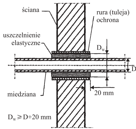
Rys. 3.2. Przykład przejścia przewodu przez strop
